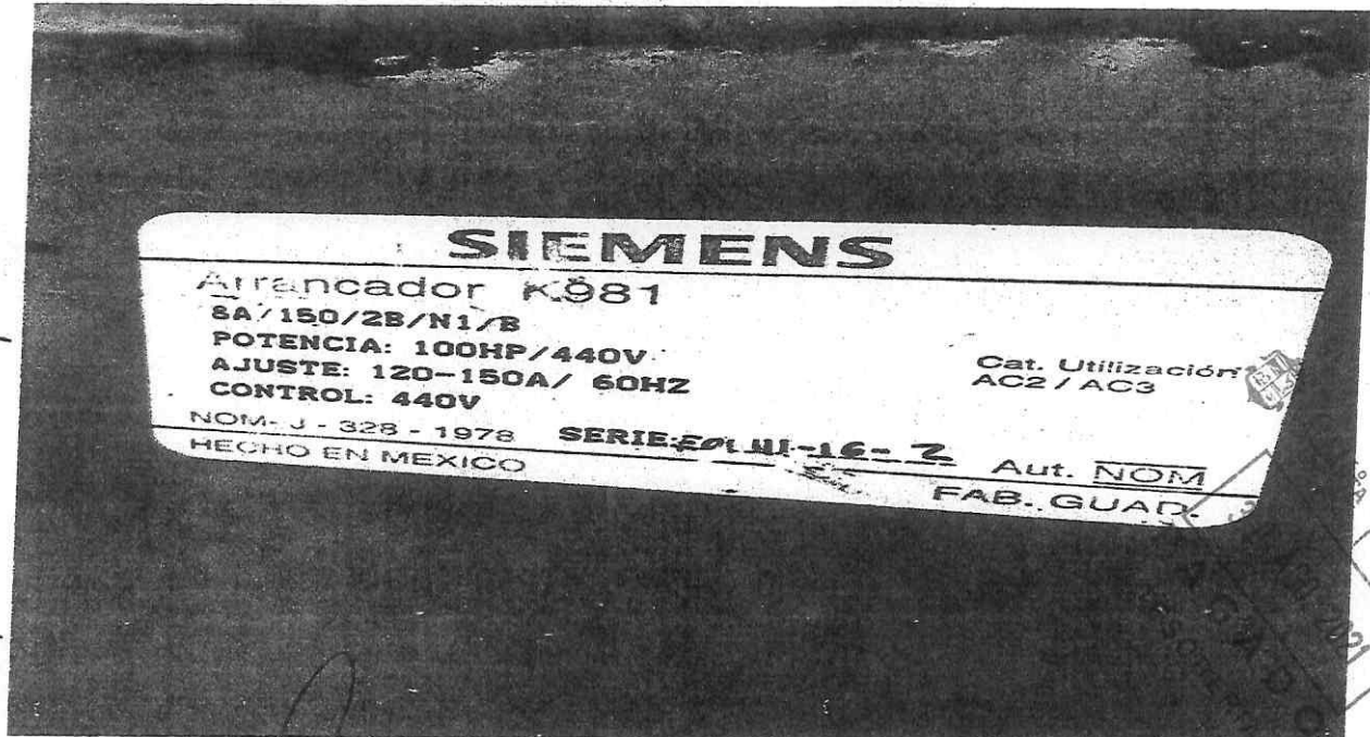
3.- Tablero de Arranque marca Siemens, Arrancador K981, de 8 o /150/2B/N1/B, Potencia de 100HP/440V, Ajuste 120-150 o / 60HZ, Cat. Utilización AC2/AC3, Control de 440V, No. De Serie E01-41-16-2, NOM- J- 328 -1978.
